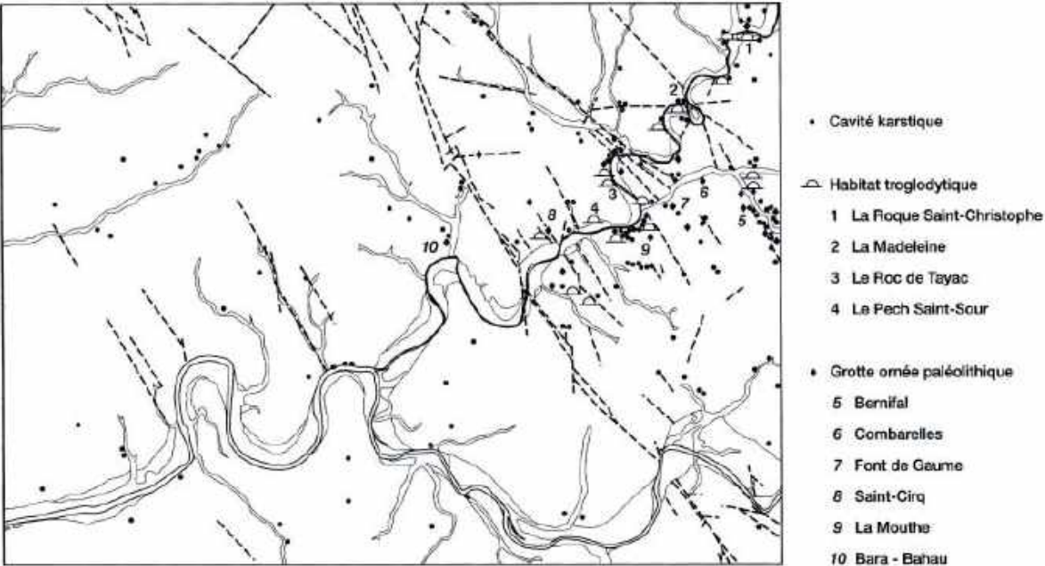
Figure 2 : Grottes ornées, habitats troglodytes et cavités de la feuille Le Bugue - doct BRGM
