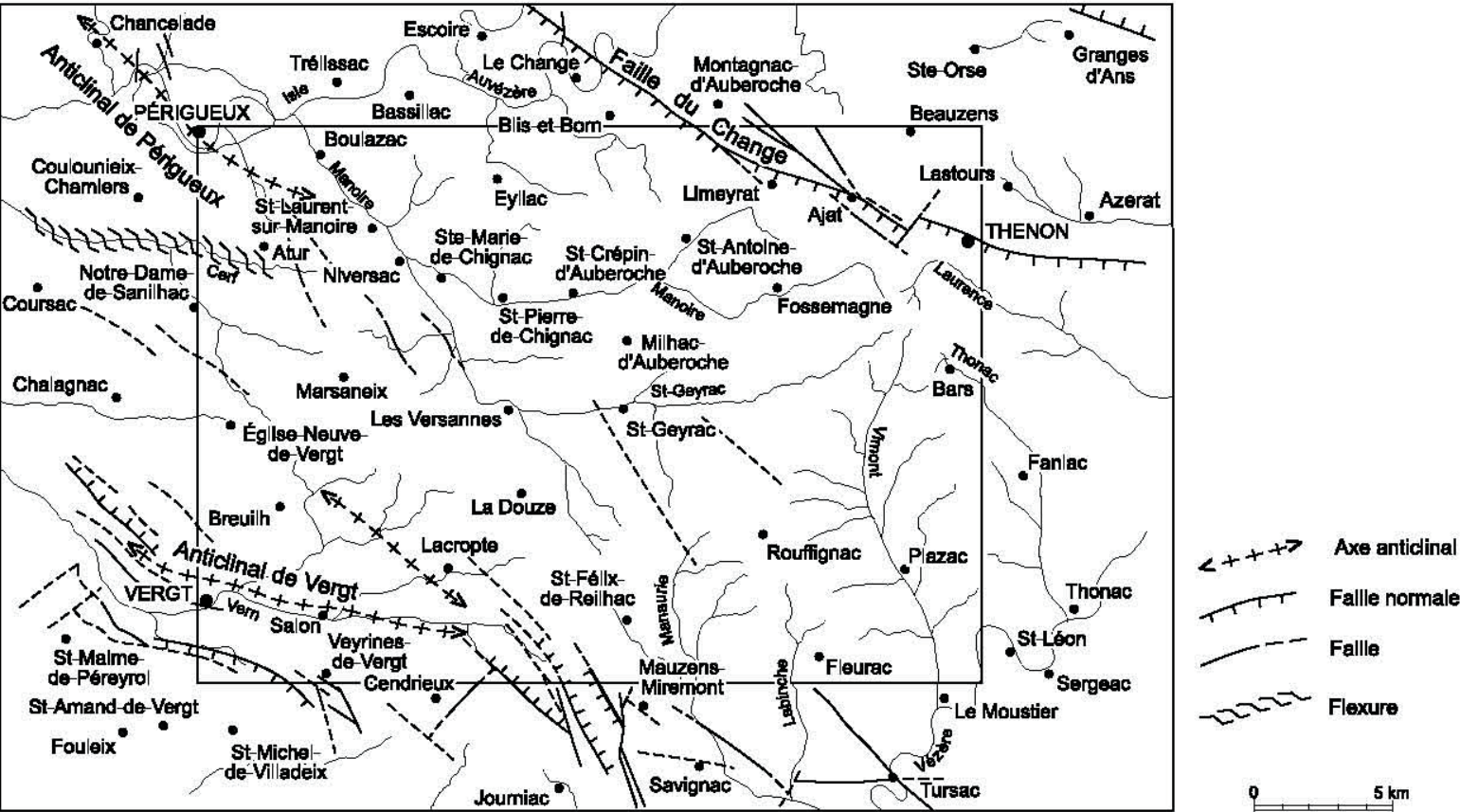
Figure 1 : Schéma structural du Périgord entre Thenon et Vergt - doct BRGM
