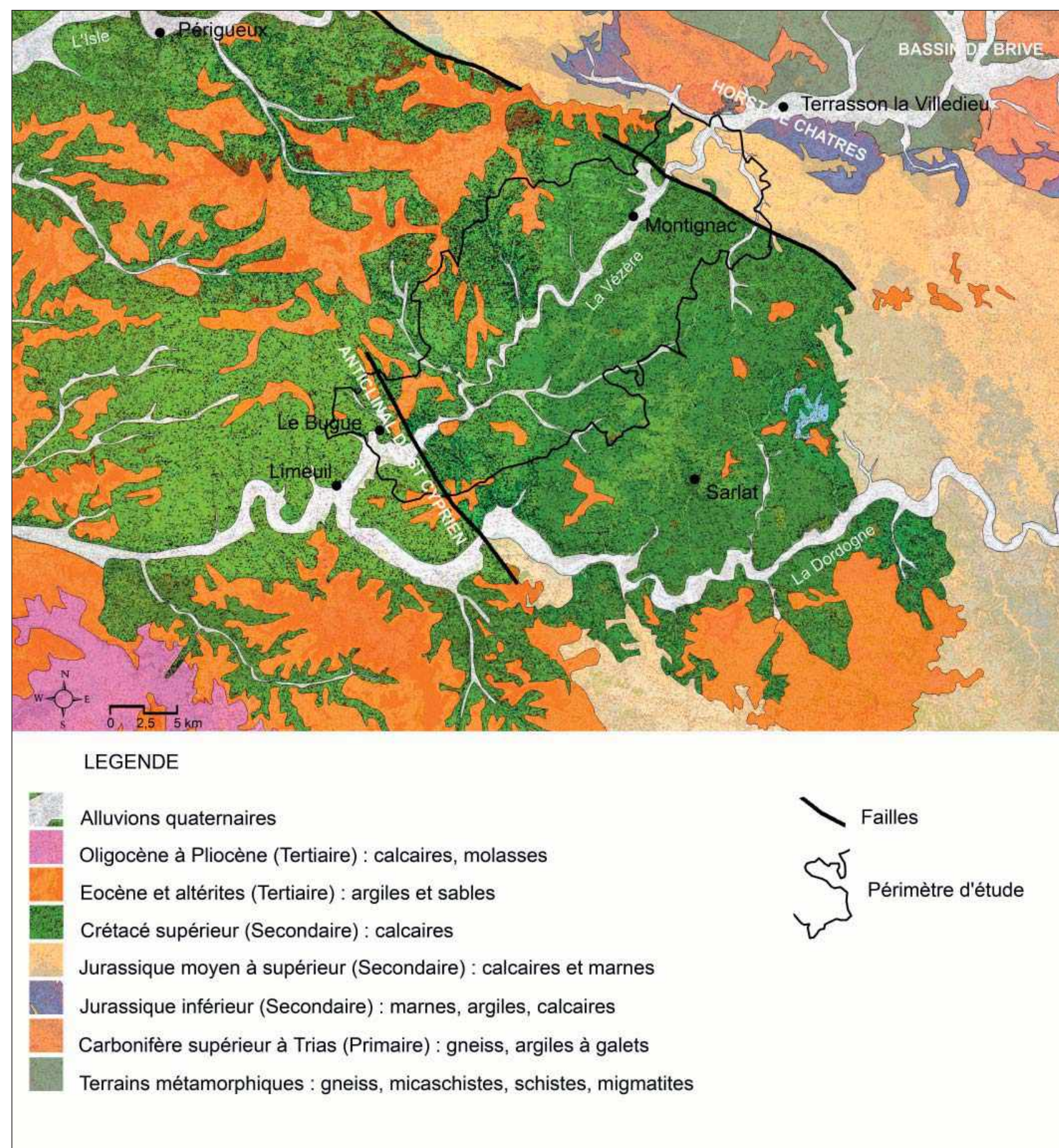
Figure 1 : Carte géologique simplifiée - interprétation des cartes du BRGM
