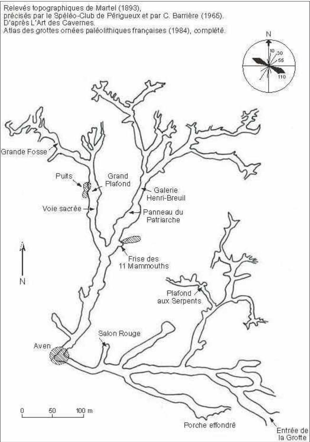
Figure 1 : Plan du réseau karstique supérieur de la grotte de Rouffignac (Croc de Grandville) et analyse structurale de la direction des galeries
