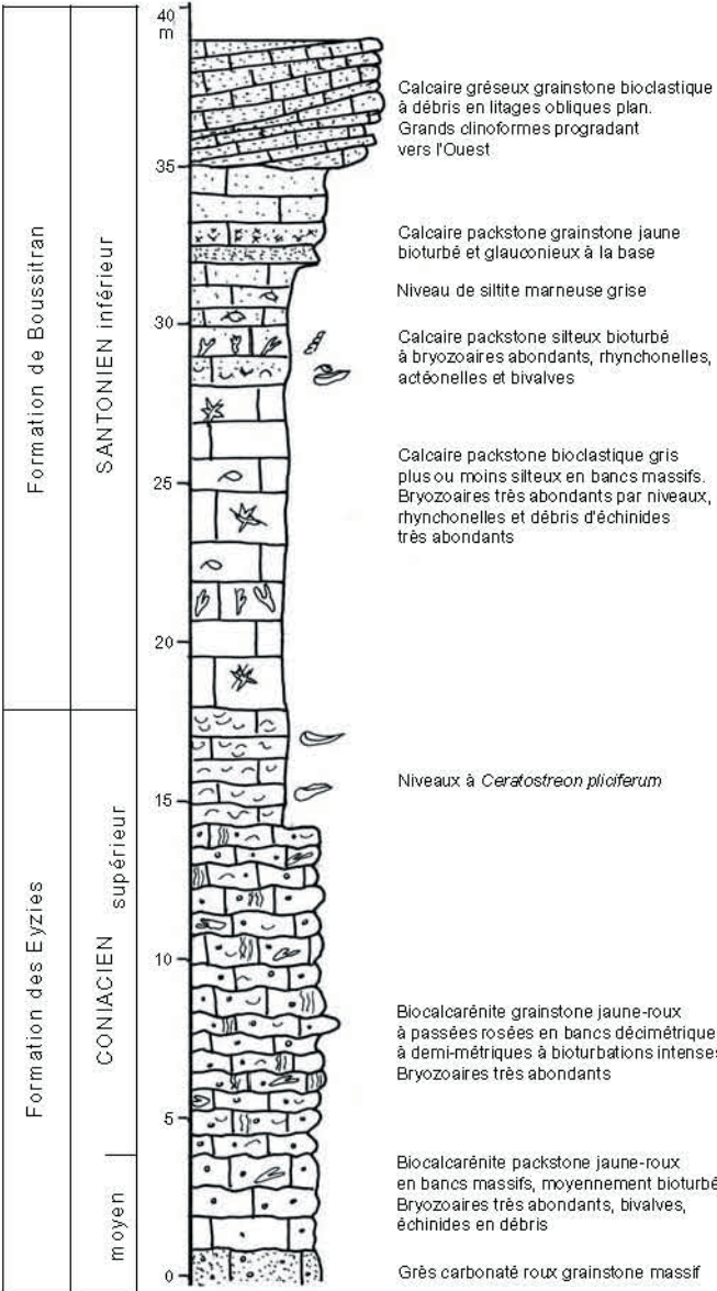
Figure 1 : Coupe du sommet de la Formation des Eyzies et de la base de la Formation de Boussitran dans la carrière de Chaban (Cote de Jord)
