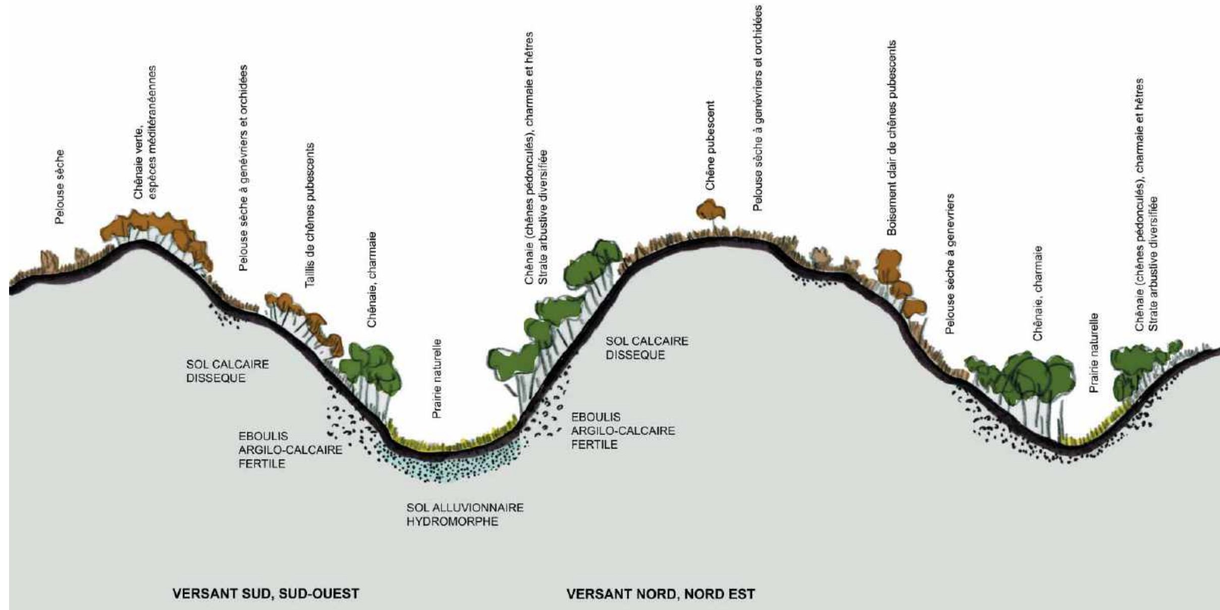
Figure 1 : Profil type d'une Combe - Etagement de la végétation naturelle (Source DOCOB - Etude BKM 2002- Relevés Mandragore)
